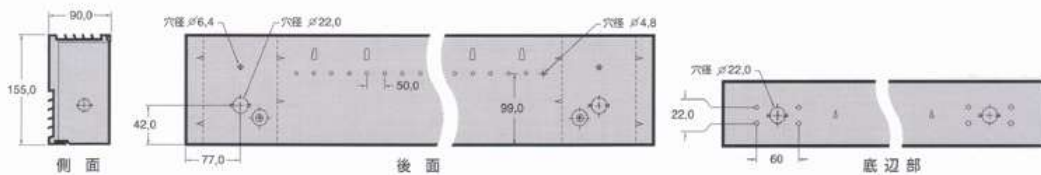
床置き用脚(オプション)
